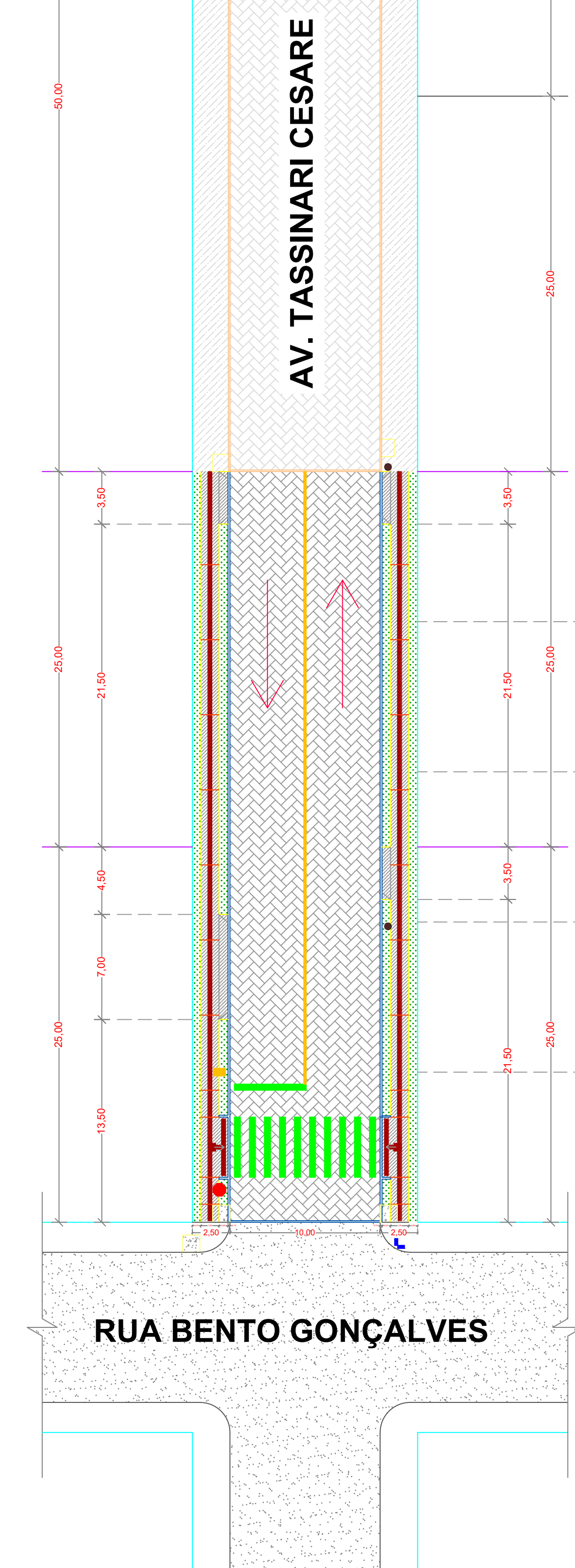
Planta Implantação e Sinalização | Escala: 1/250
