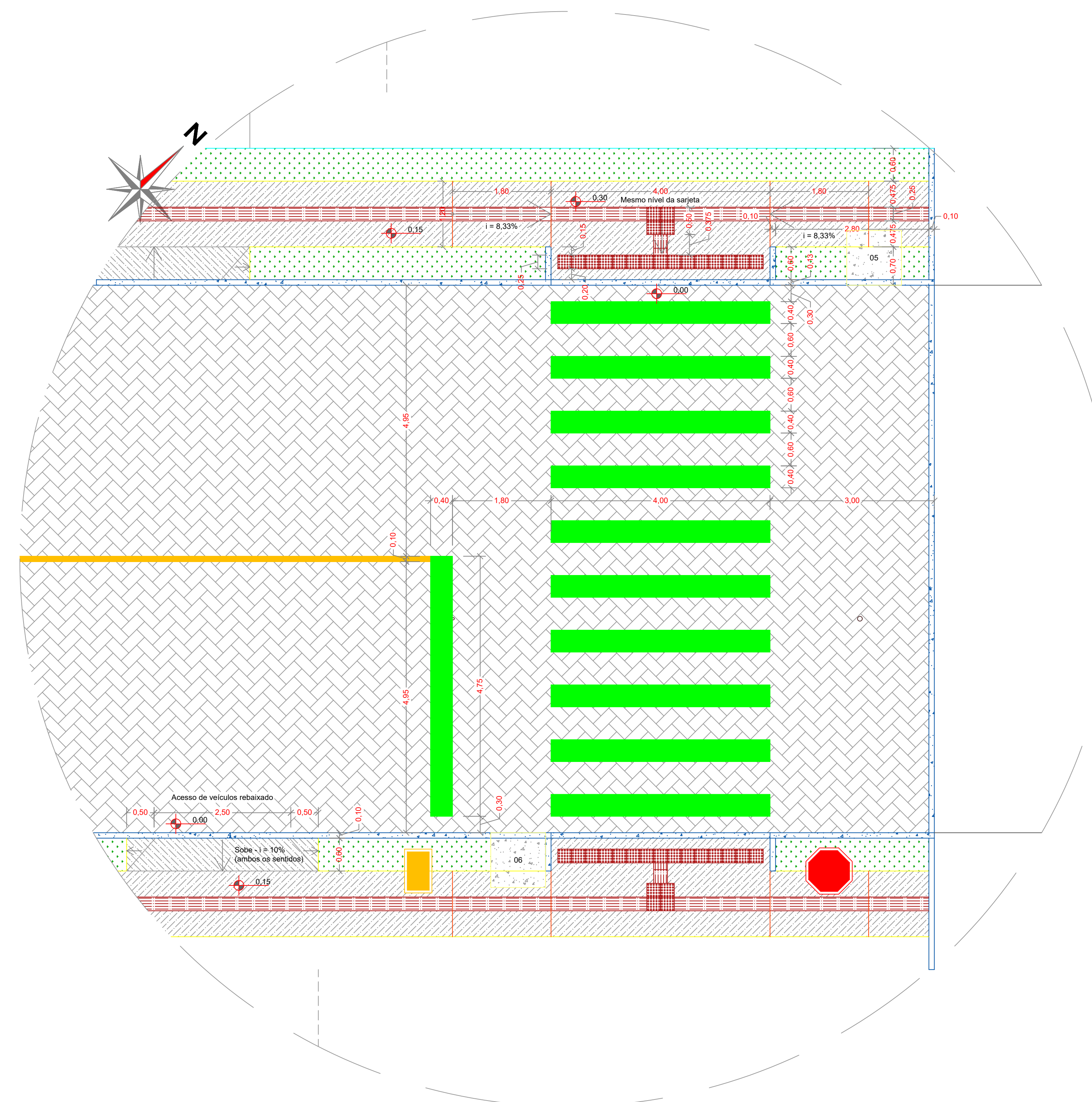
DETALHE 01 - Travessia para pedestres em via pública | Escala 1/50
