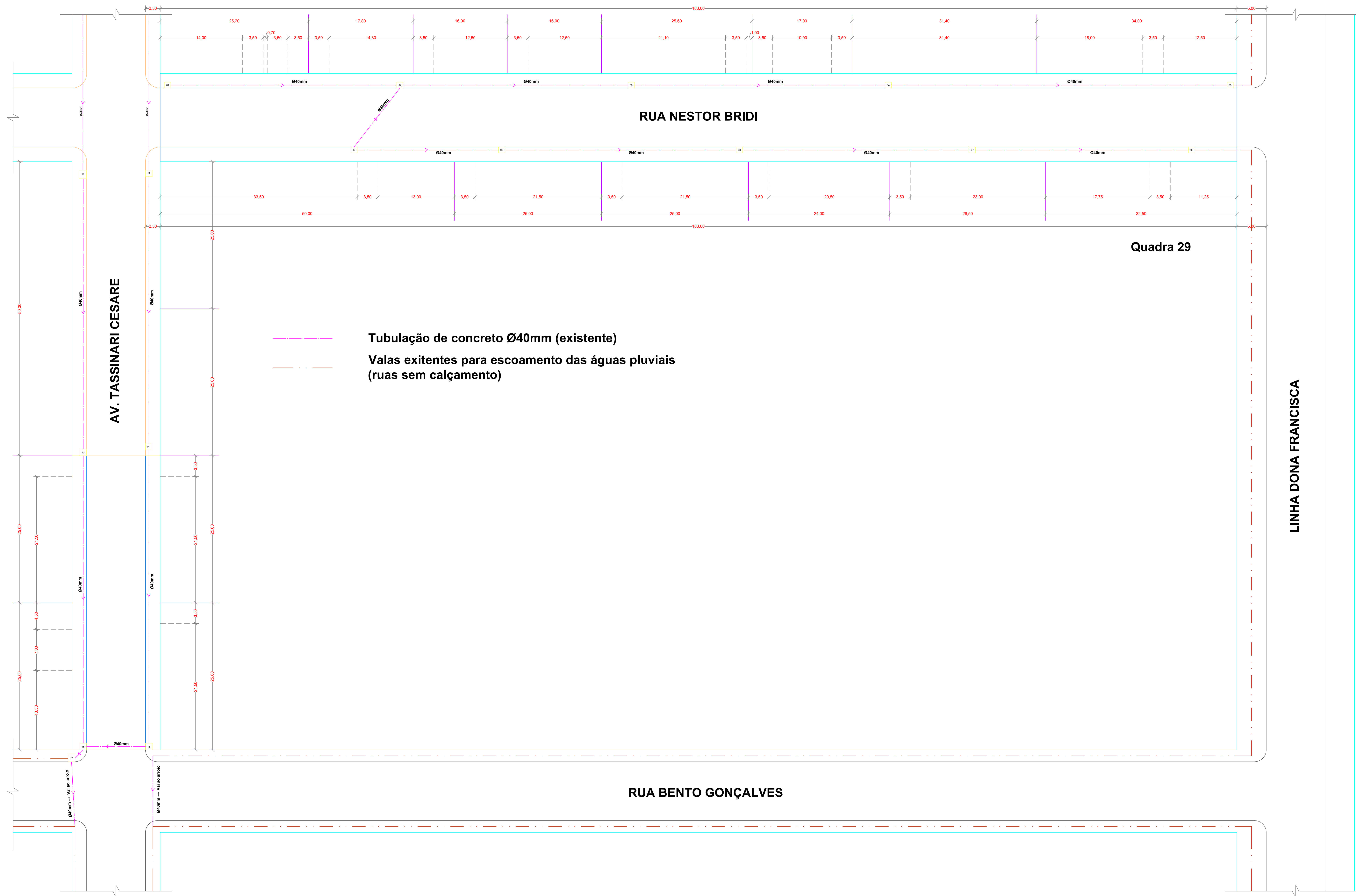
Planta Locação Rede Esgoto Pluvial | Escala: 1/250
